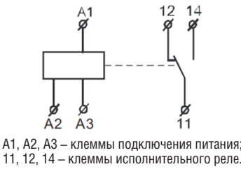
Рисунок Б.2 – Электрическая схема реле с напряжением катушки 230В AC и 24В AC/DC и 1-м выходом
