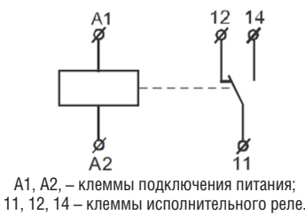
Рисунок Б.1 – Электрическая схема реле с напряжением катушки 24В AC/DC и 1-м выходом
