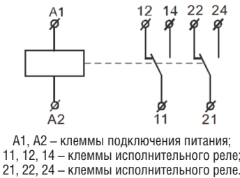
Рисунок Б.3 – Электрическая схема реле с напряжением катушки 24В AC/DC и 2-мя выходами
