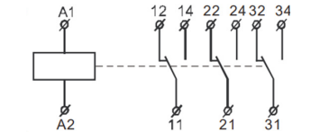
Рисунок Б.5 – Электрическая схема реле с напряжением катушки 230В AC и 24В AC/DC и 3-я выходами
