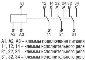
Рисунок Б.5 – Электрическая схема реле с напряжением катушки 230В AC и 24В AC/DC и 3-я выходами
