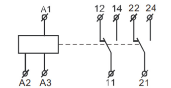
Рисунок Б.4 – Электрическая схема реле с напряжением катушки 230В AC и 24В AC/DC и 2-я выходами
