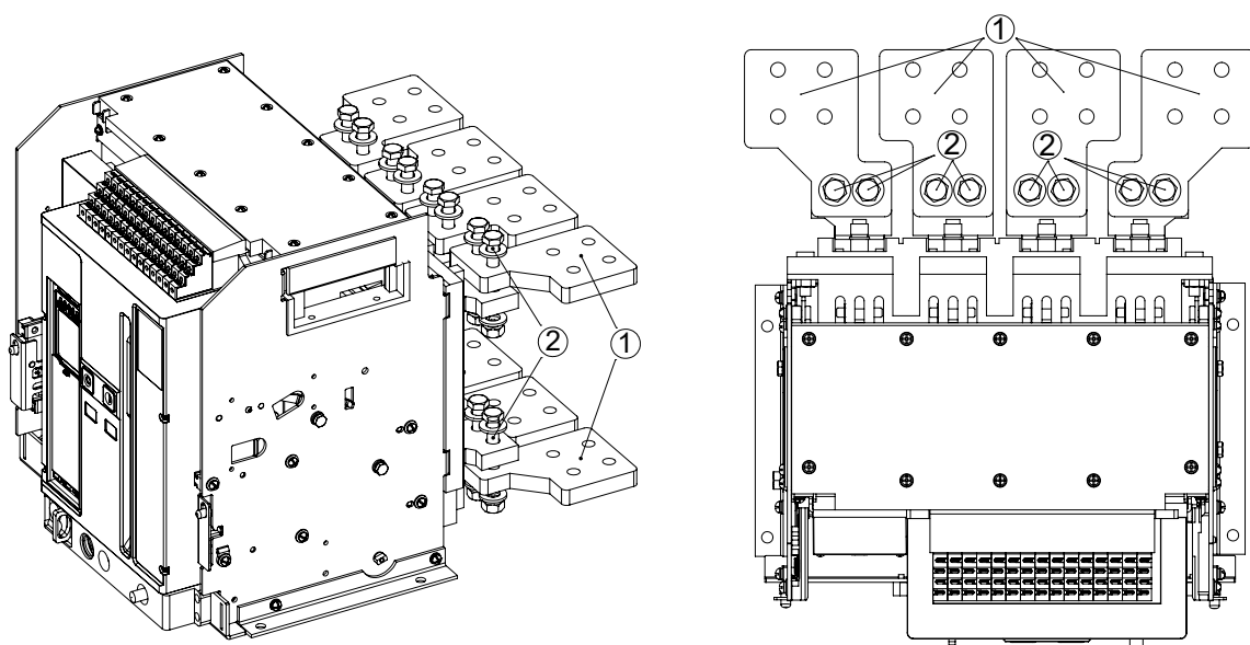
Рисунок 2 – Установка комплекта расширителей на четырёхполюсный выключатель 1-Расширители выводов, 2-Крепление
