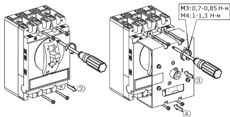
Рисунок 3 – Установка стержня поворотной рукоятки
