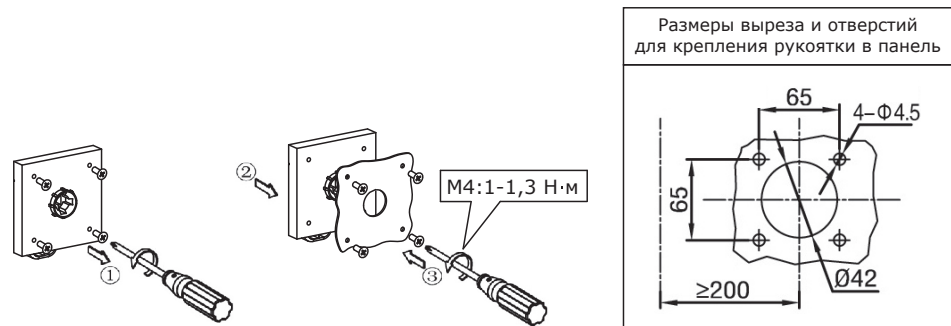
Рисунок 4 – Установка рукоятки
