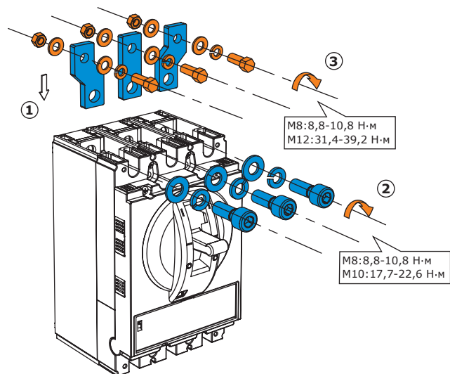
Рисунок 1 – Монтаж выводов расширенных
