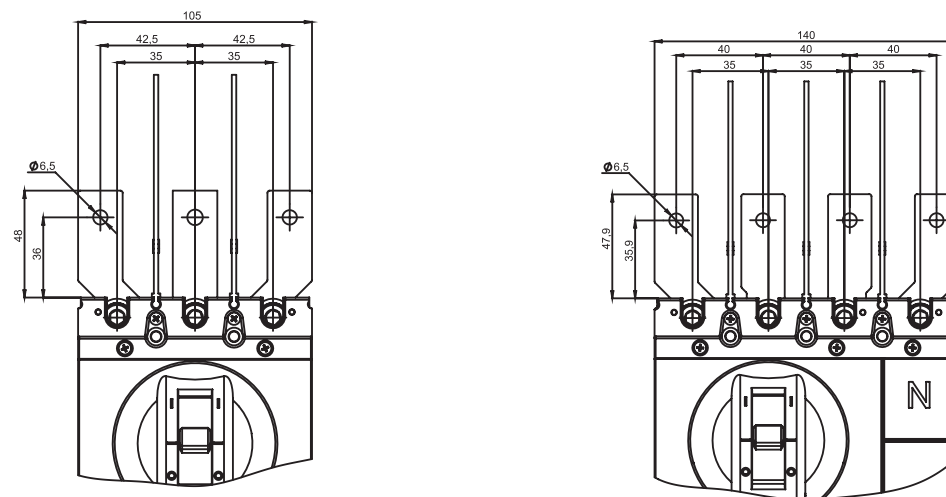
Рисунок 3 – Габаритный чертеж выводов расширенных OptiMat T250 3p, OptiMat T250 4p
