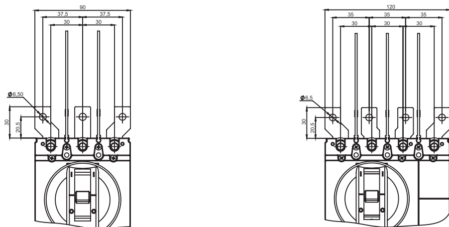
Рисунок 2 – Габаритный чертеж выводов расширенных OptiMat T125-T160 3p, OptiMat T125-T160 4p
