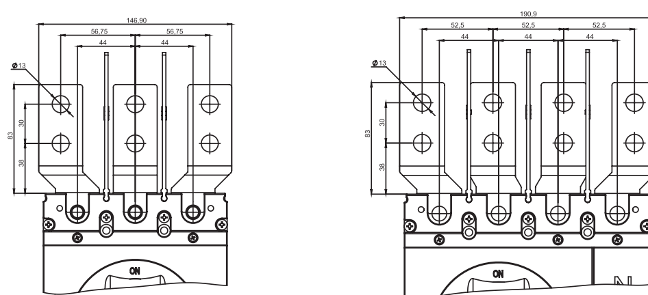
Рисунок 4 – Габаритный чертеж выводов расширенных OptiMat T400-T630 3p, OptiMat T400-T630 4p,
