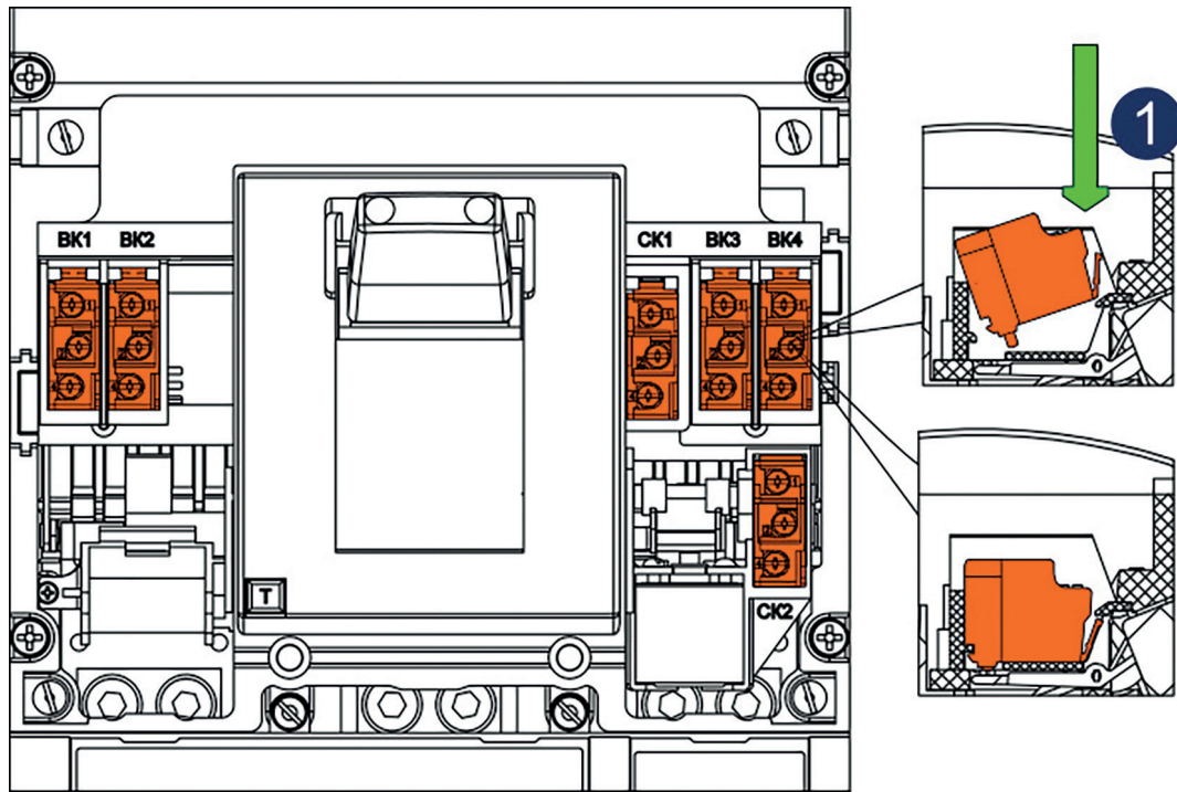
Рисунок 10 – Установка вспомогательных контактов OptiMat D800, D1000, D1250, D1600.
