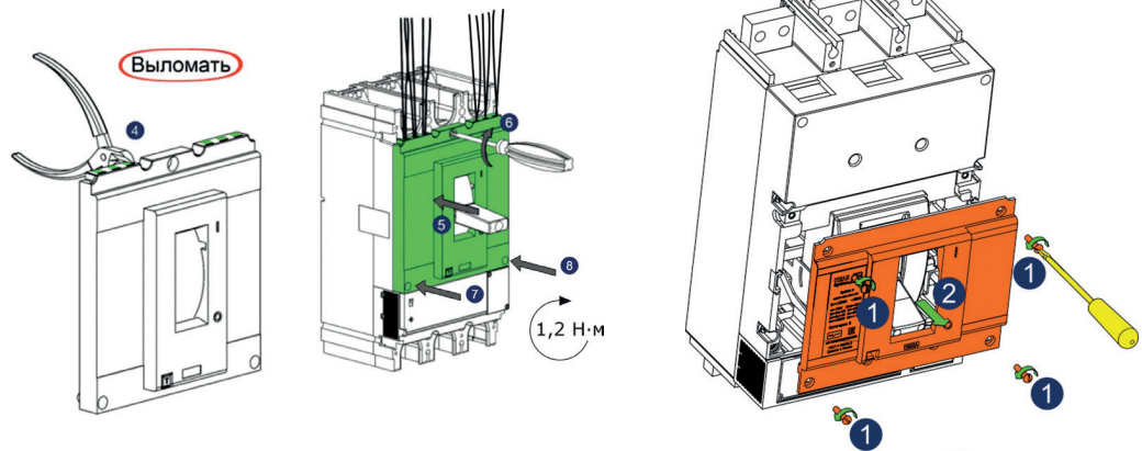
Рисунок 10 – Установка вспомогательных контактов OptiMat D800, D1000, D1250, D1600.
