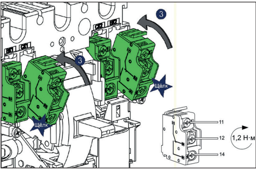
Рисунок 2 – Установка вспомогательных контактов OptiMat D100, D160, D250.
