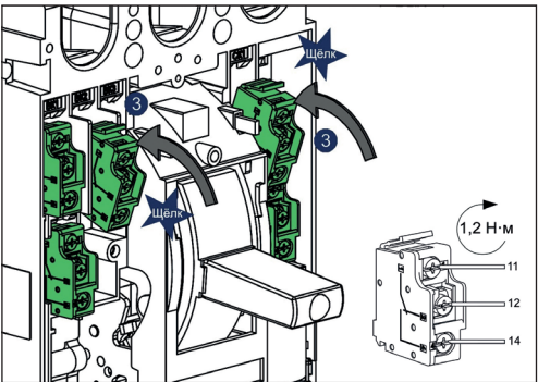
Рисунок 7 – Установка вспомогательных контактов OptiMat D400, D630.
