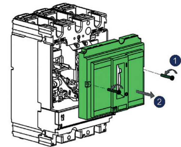
Рисунок 2 – Установка вспомогательных контактов OptiMat D100, D160, D250.
