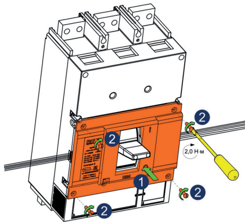
Рисунок 11 – Установка крышки маркировочной OptiMat D800, D1000, D1250, D1600 и пример вывода проводов.
