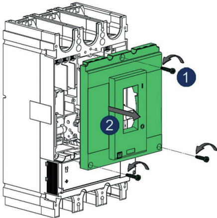
Рисунок 7 – Установка вспомогательных контактов OptiMat D400, D630.
