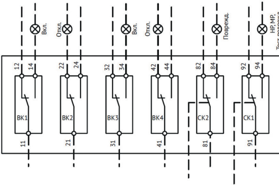
Рисунок 6 – Электрическая схема вспомогательных контактов ВК/СК1/СК2 OptiMat D400, D630
