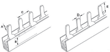
Шина типа PIN 2P 63, 100 A
