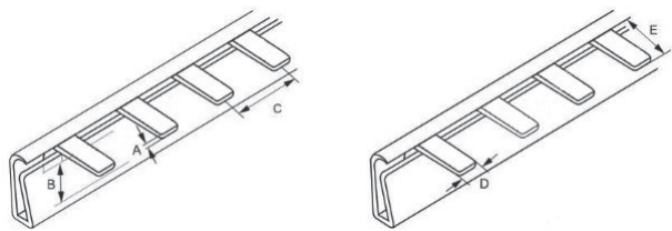
Шина типа PIN 1P 63, 100 A
