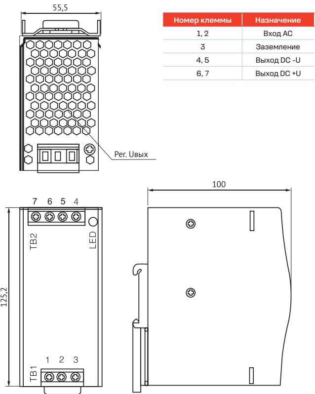
Блок питания DR-75
