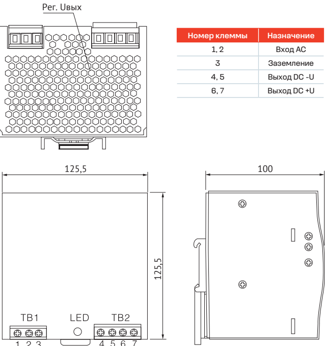
Блок питания DR-240
