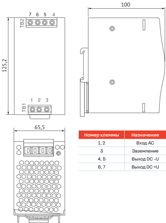
Блок питания DR-120
