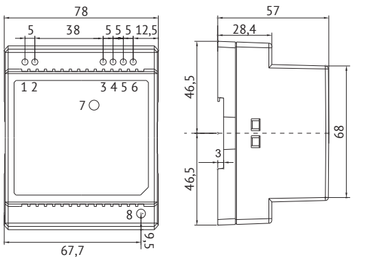
Блок питания DR-30, 45, 60
