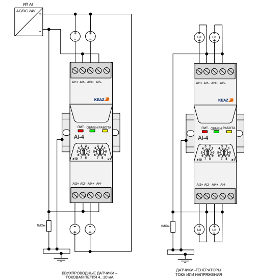
Рисунок 3 — Схемы подключения модуля
