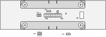
Рисунок 2 — Расположение перемычек XP2 и XP3
