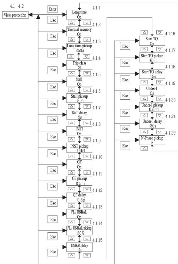
Рисунок 4 – Интерфейс меню View dial protection (Просмотр ручных уставок) или View electron protection (Просмотр электронных уставок)
