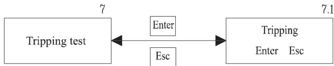
Рисунок 11 – Интерфейс меню Tripping test (Тест срабатывания)
