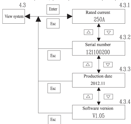
Рисунок 5 – Интерфейс меню View system (Просмотр системных параметров)
