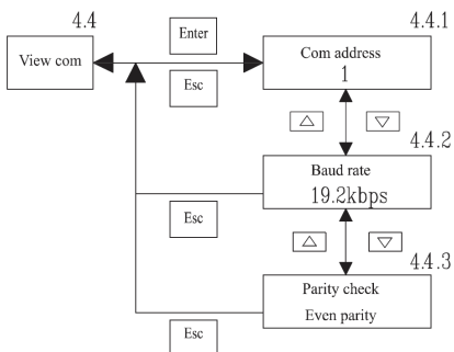
Рисунок 6 – Интерфейс меню View com (Просмотр параметров связи)
