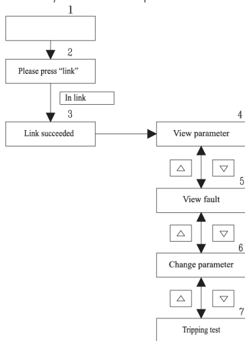
Рисунок 2 – Навигация по основному меню блока тестирования ET TEST
