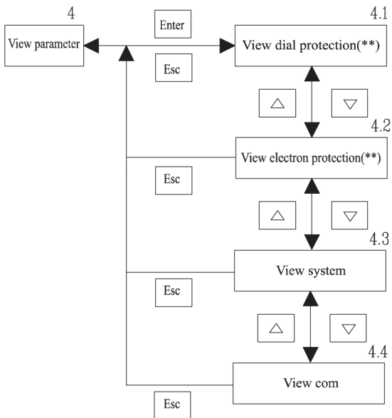
Рисунок 3 – Интерфейс меню View parameter (Просмотр параметров)
