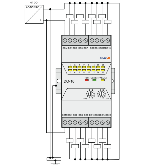
Рисунок 3 — Схемы подключения модуля
