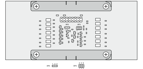
Рисунок 2 — Расположение перемычек XP2 и XP3
