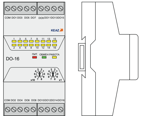
Рисунок 1 — Внешний вид модуля
