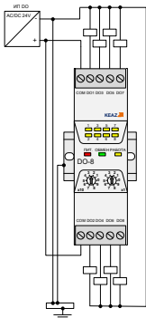
Рисунок 3 — Схемы подключения модуля
