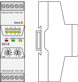
Рисунок 1 — Внешний вид модуля
