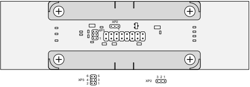
Рисунок 2 — Расположение перемычек XP2 и XP3
