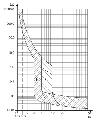
Рисунок Б.1 – Защитные характеристики В, С в цепи переменного тока при контрольной температуре плюс 30 °С
