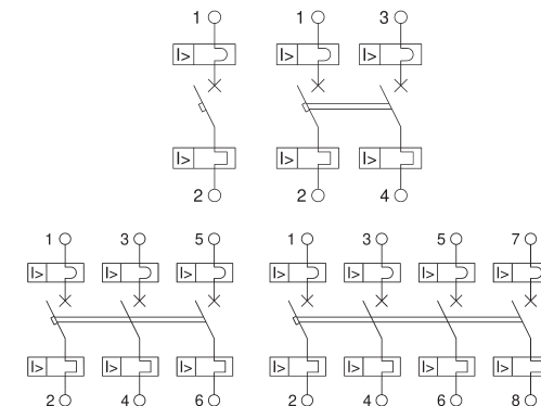
Рисунок Г.1 – Принципиальные электрические схемы выключателей
