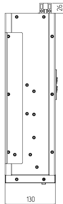
Рисунок А.3 — Габаритный чертеж OptiSine 30K-15A-W3, OptiSine 30K-15A-W4, размеры в мм
