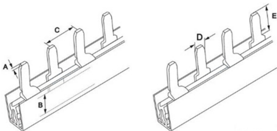
Рисунок 6 – Шина типа PIN 2P 63, 100 А
