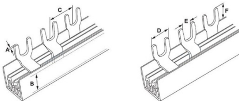
Рисунок 3 – Шина типа FORK 3P 63, 100 А
