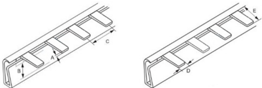
Рисунок 5 – Шина типа PIN 1P 63, 100 А
