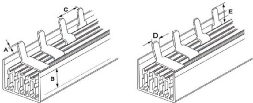
Рисунок 8 – Шина типа PIN 4P 63, 100 А
