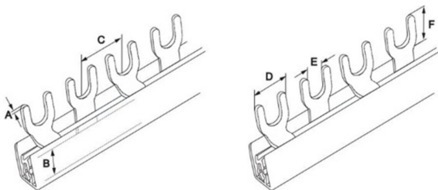
Рисунок 2 — Шина типа FORK 2P 63, 100 А
