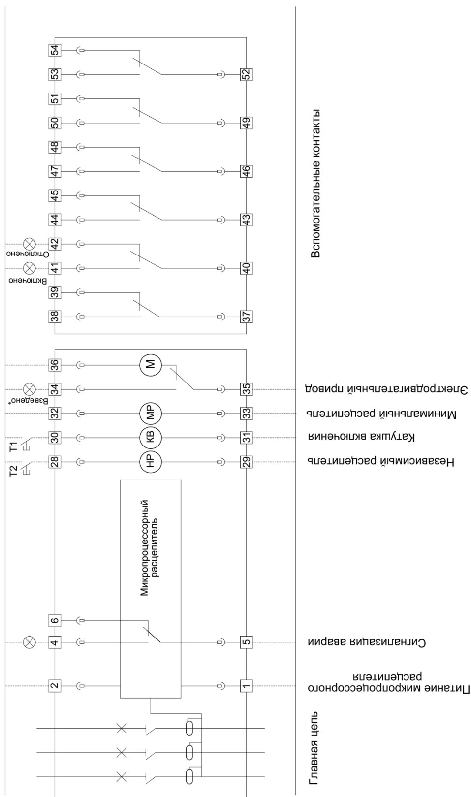
Рисунок Б.1 - Схема электрическая принципиальная выключателя OptiMat A630-1600-S1 с электронным расцепителем MR5.0
