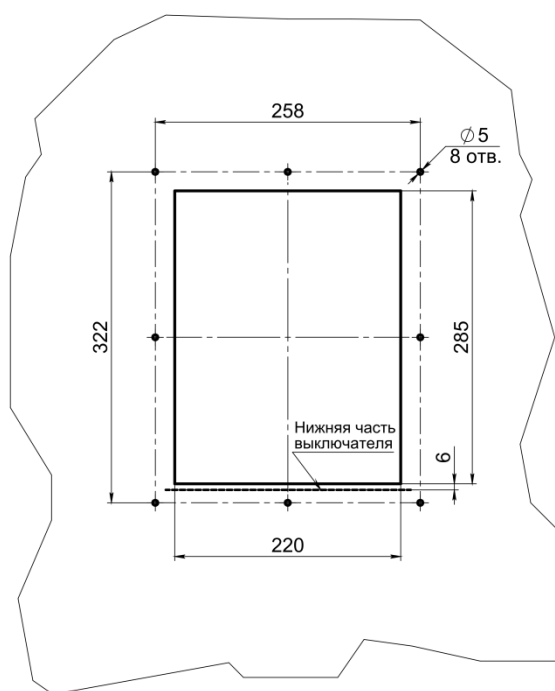
Рисунок А.4 – Вырез в дверце для автоматического выключателя OptiMat A630-1600-S1 стационарного исполнения
