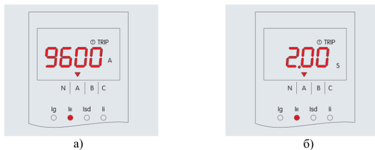
а) ток срабатывания; б) время срабатывания. Рисунок 7
