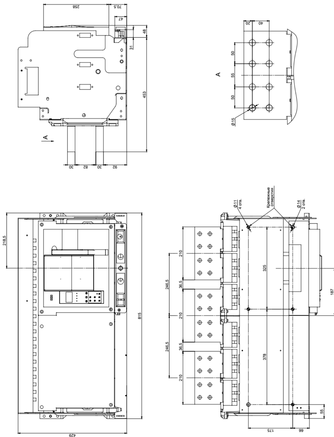
Рисунок А.9 – Автоматический выключатель OptiMat A5000-S5 выдвижного исполнения на номинальный ток 5000 А (120 кА)
