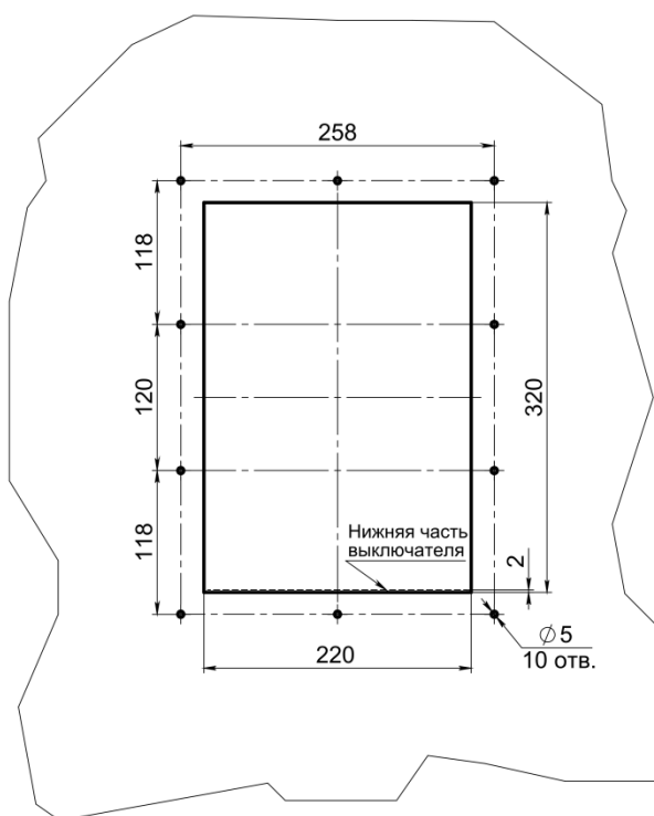
Рисунок А.8 – Вырез в дверце для автоматического выключателя OptiMat A630-1600-S1 выдвижного исполнения
