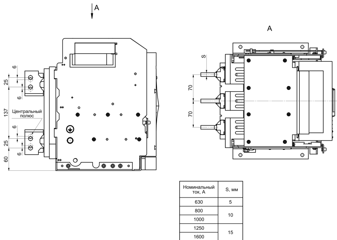
Рисунок А.7 – Автоматический выключатель OptiMat A630-1600-S1 выдвижного исполнения на номинальные токи 630 – 1600 А с вертикальным расположением Выводов
