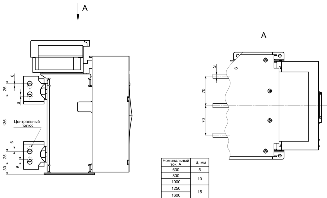
Рисунок А.3 – Автоматический выключатель OptiMat A630-1600-S1 стационарного исполнения на номинальные токи 630 – 1600 А с вертикальным расположением выводов
